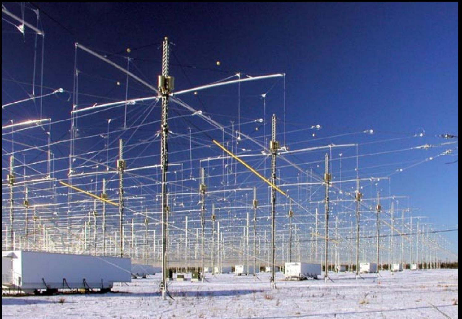
Campos típicos de antena HAARP KW
